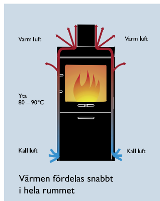
Konvektion
